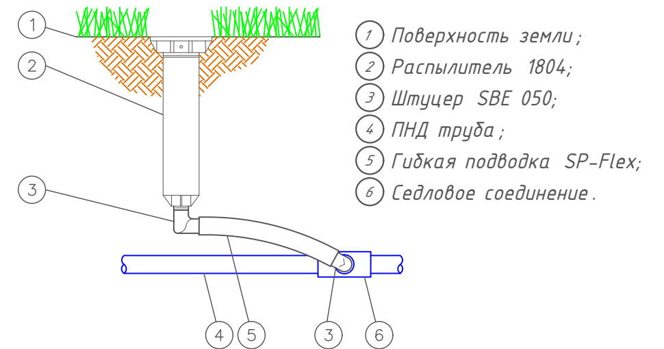
Схема подключения распылителя 1804
